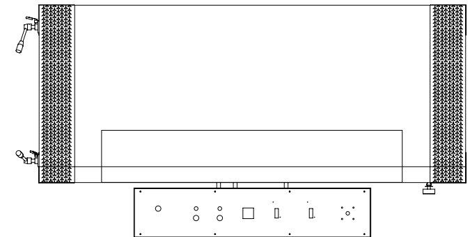
Planta /Top
