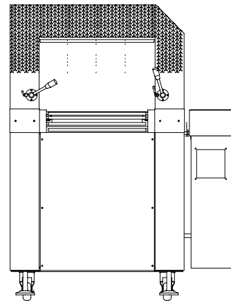
Perfil /Side
