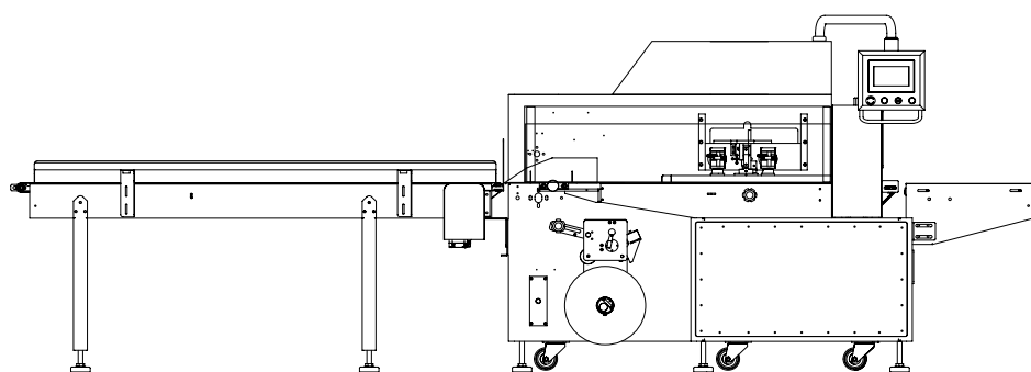
Alzado /Front
