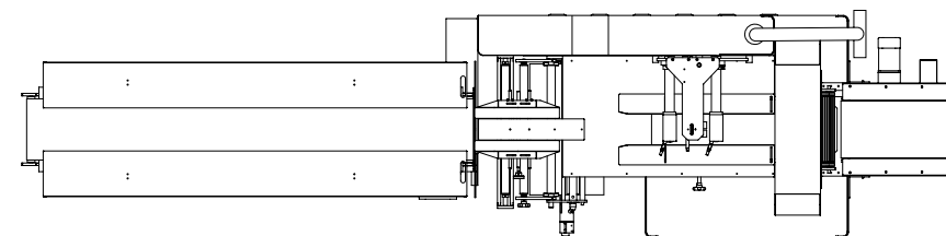
Planta /Top
