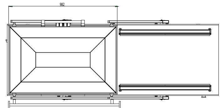
Planta /Top
