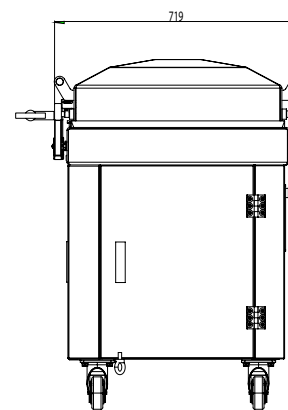
Perfil /Side
