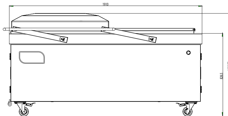
Alzado /Front
