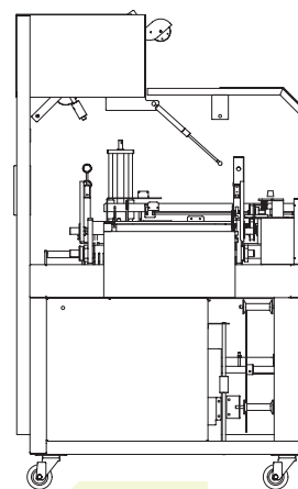
Perfil /Side
