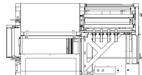
Planta /Top
