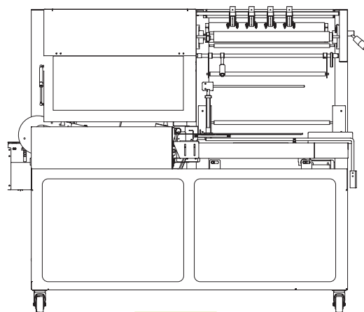
Alzado /Front
