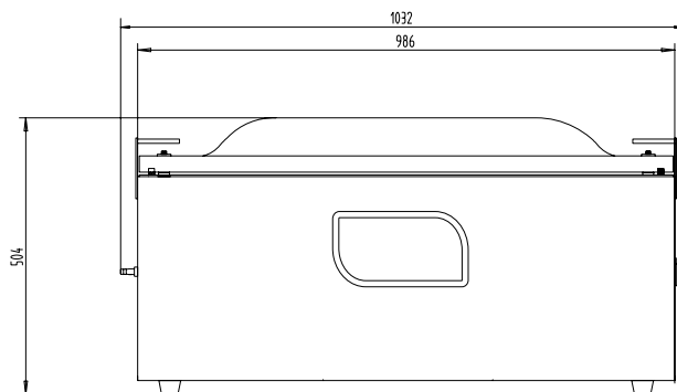
Alzado /Front
