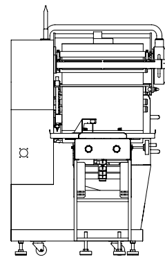
Perfil /Side
