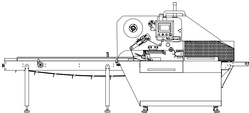
Alzado /Front
