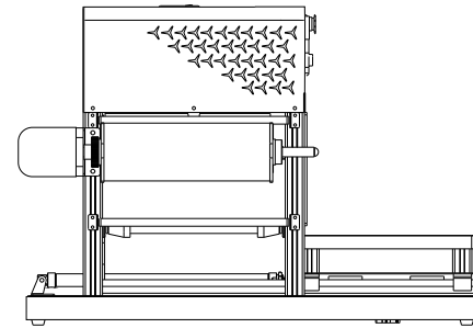
Alzado /Front
