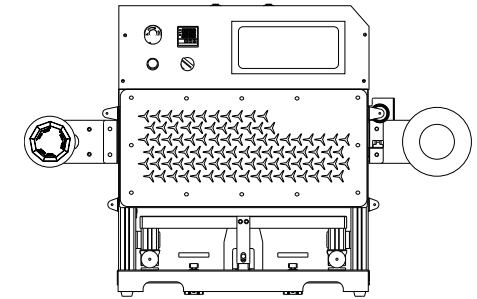
Perfil /Side
