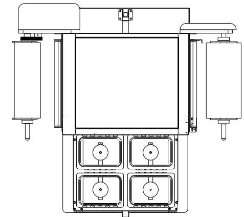
Planta /Top
